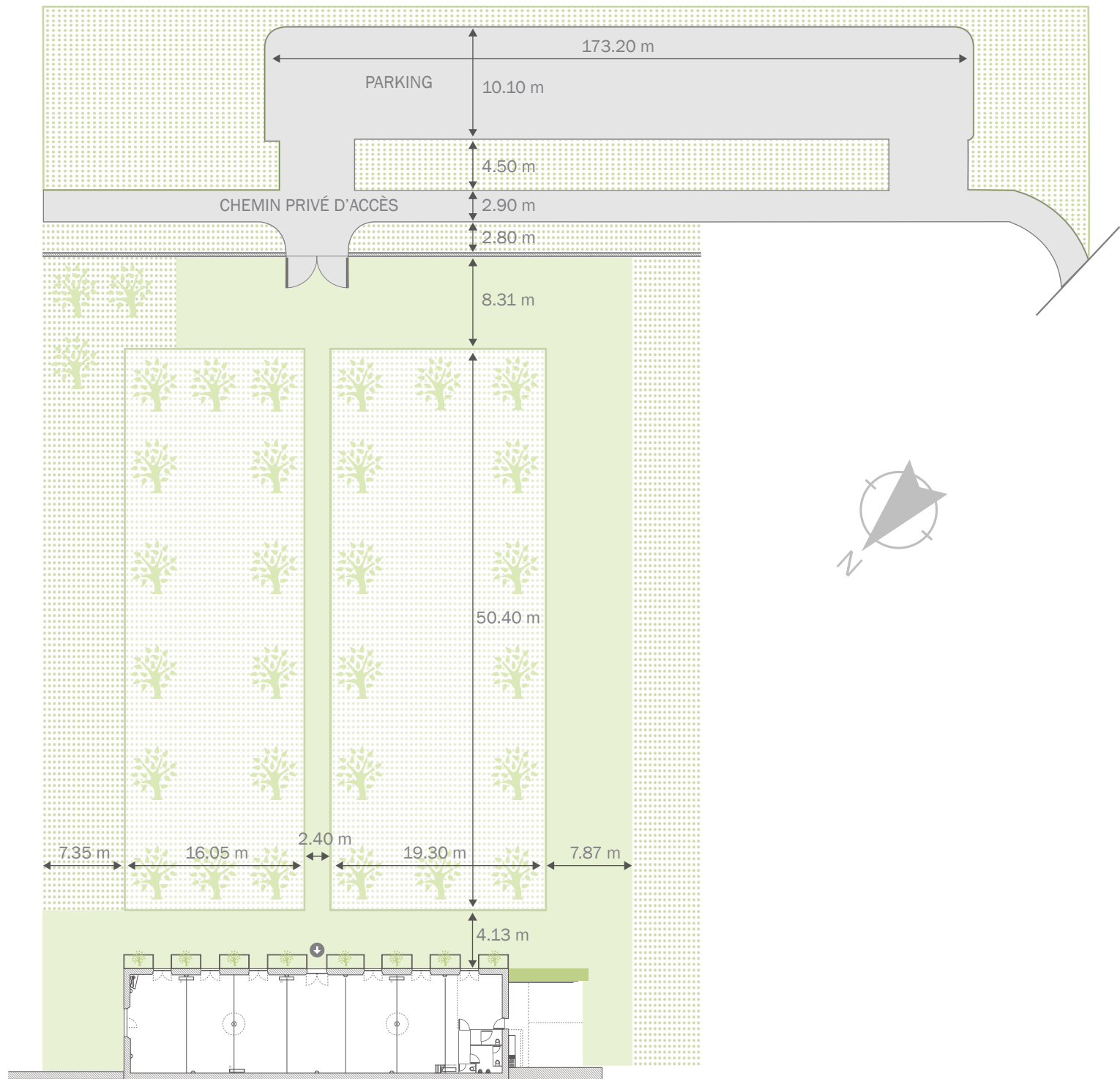
PLAN DE MASSE - Éch : 1/100 ème
